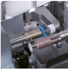
ES-versa的标准切割系统可进行粗加工、尖边、抛光、开槽和安全边切削。
