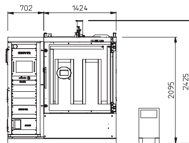
前视图
